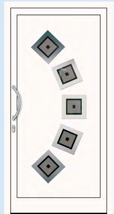
Kunststoff Modell 2078 (PG30) Aluminium Modell 4078 (PG32) beidseitig Edelstahlrahmen Glas: Klar plan, Mattierung „Madrid“ Griff: HA1049 Edelstahl PZ-Rosette: HA1075 Edelstahl (oval)
