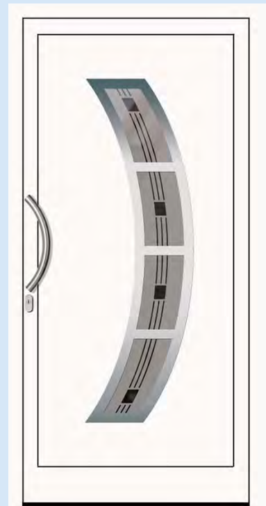
Kunststoff Modell 2012 (PG32) Aluminium Modell 40112 (PG33) Beidseitig Edelstahlrahmen Glas: Iso klar, Mattierung „Alexandria“ Griff: HA1061 Edelstahl PZ-Rosette: HA1077 Edelstahl mit Kernziehschutz
